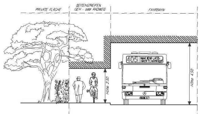
Freizuhaltendes Lichtraumprofil an öffentlichen Straßen, Wegen und Plätzen
